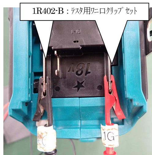
図 1-3 ワニ口クリップ取付
