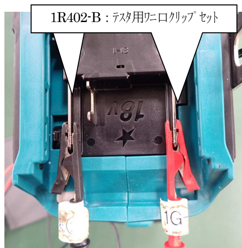
図 1-3 ワニクリップ取付
